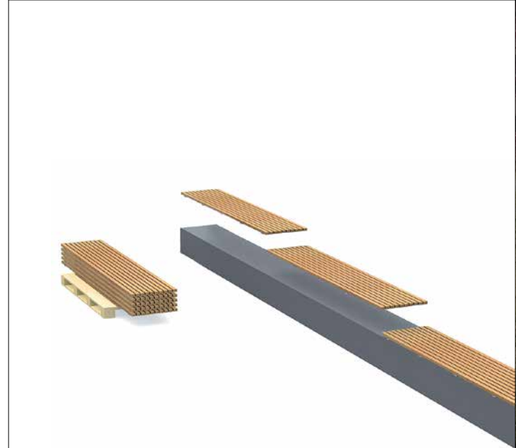
Le module à lattes préfabriquées Wood Top est doté d'une version miniature des peignes Streetlock®. En option, avec des moulures verticales.
